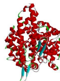
Gambar 4. Struktur ACE
